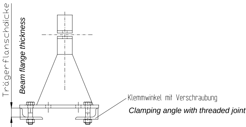
Abb. 3 : Trägerklemmbefestigung bei Befestigungsform A und C
