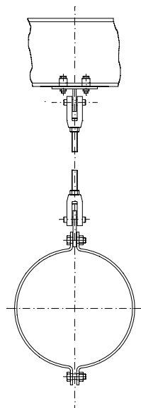
Abb. 1: a) Rohrleitung quer zum Trägerprofil Figure 1: a) pipe cross to the beam
