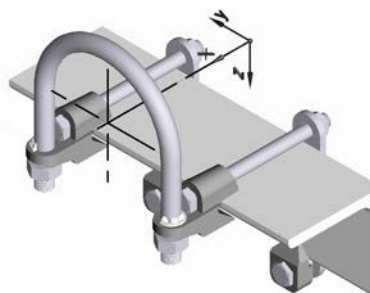
Gleitlager DN 100 auf Trägerprofil L 100 x 10
