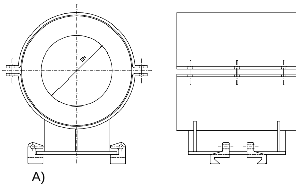
Abb. 9 : A) Vorisiertes Rohrlager mit Klemmsystem als Führungslager mit Abhebesicherung (FLA) B) Vorisiertes Rohrlager mit Klemmsystem als Führungslager (FL)
