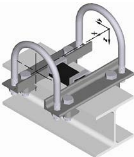
Festpunktlager DN 100 auf Trägerprofil HEB100
