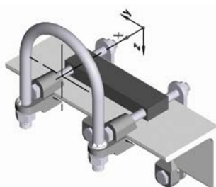
Gleitlager DN 100 auf Trägerprofil L 100 x 10
