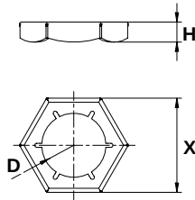
Bestellbeispiel / order example: PAL M12 galverz / cold-galvanized
