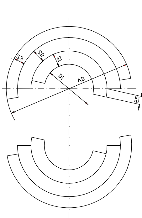
Abb. 3 : Aufbau einer dreilagigen Isolierschale
