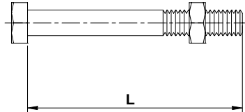
Bestellbeispiel / order example: DIN 601 M12 4.6 L=? galverz / cold-galvanized
