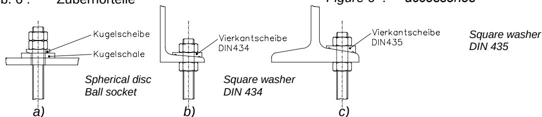
Abb. 6 : Zubehörteile
