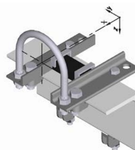
Gleitlager DN 100 auf Trägerprofil L 150 x 100 x 10
