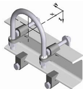
Gleitlager DN 100 auf Trägerprofil UNP 100
