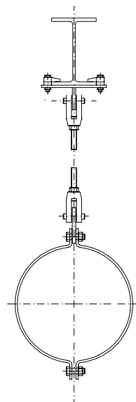
b) Rohrleitung parallel zum Trägerprofil b) pipe parallel to the beam
